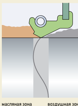
Уплотнительная кромка SKF WAVE с синусоидальной рабочей частью
