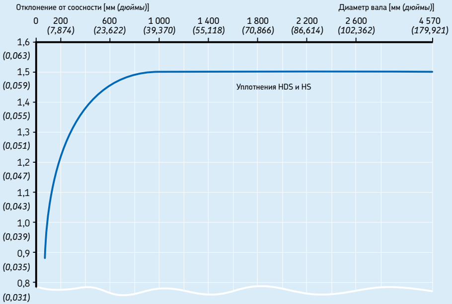
Максимальное допустимое отклонение от соосности в зависимости от диаметра вала
