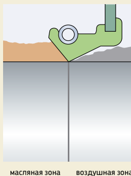
Стандартная уплотнительная кромка с прямым профилем
