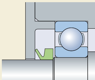
V-образное уплотнение
