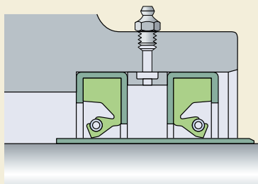
Дистанционное кольцо и пресс-маслёнка
