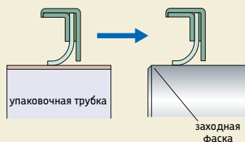
б) Монтаж по направлению кромки из PTFE
